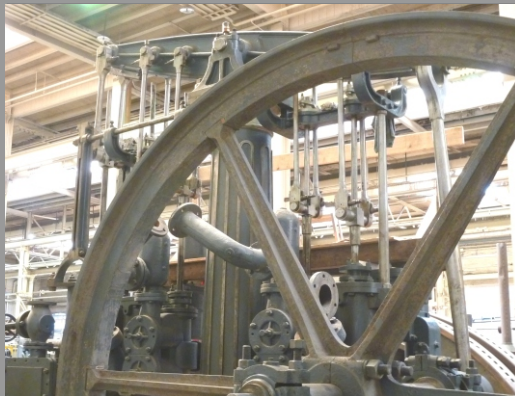
1-Zylinder Balancier-Dampfmaschine Giesserei und Maschinenfabrik Berlin 1859 Wasserwerk Berlin, Technorama
