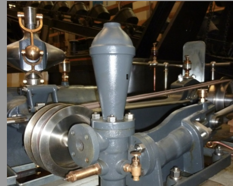
1-Zylinder- Dampfmaschine Sulzer, Winterthur 1890 Molkereifachschule Rütli, Zollikofen BE
