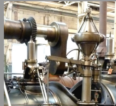
2-Zylinder-Ventildampfmaschine Sulzer, Winterthur 1902 Tram Basel, Müller Strengelbach AG
