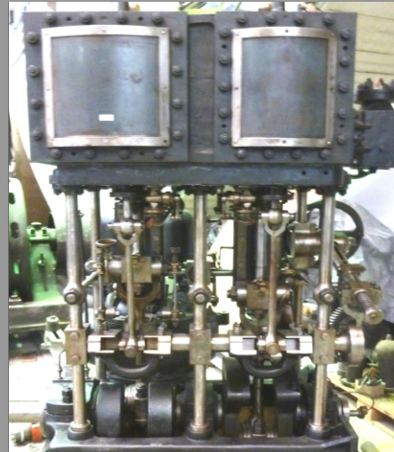
2-Zylinder Schiffsdampfmaschine Escher Wyss, Zürich 1910 DS «Lützelau», Zürichsee, Technorama
