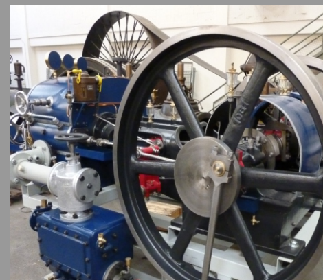
2 Zylinder-Dampfmaschine Assmann + Stockder, Stuttgart 1920 Labormaschine, Technikum Biel
