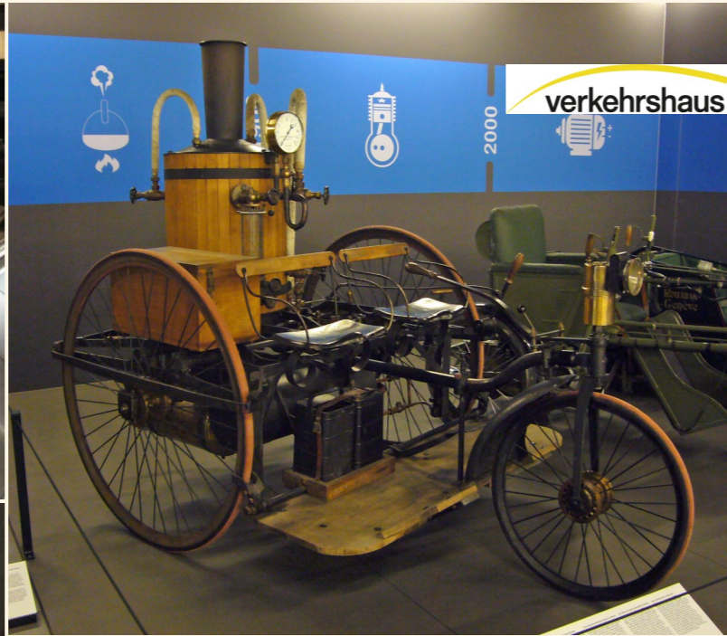
Eines der ältesten Autos der Schweiz Dampf-Dreirad gebaut von der SLM 1887
