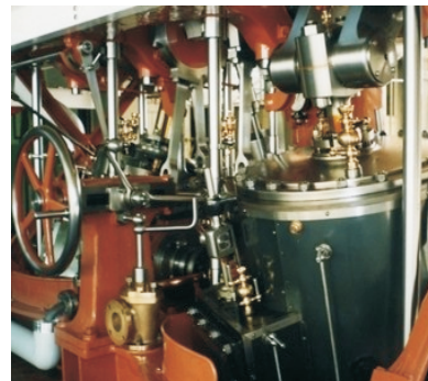
1899 Schiffsdampfmaschine 2-Zylinder Verbund-Dampfmaschine Escher Wyss, Zürich
